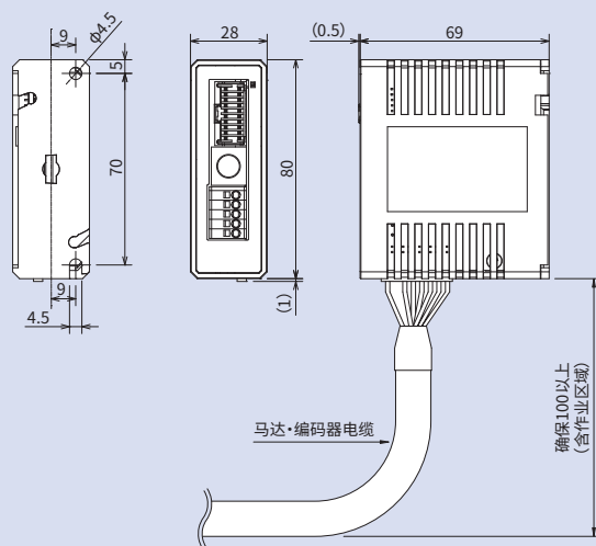
[螺丝固定安装规格]
